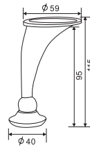
FF2018CP MATERIAL: Zinc Alloy
