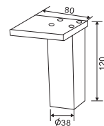
FF2024CP MATERIAL: Steel
